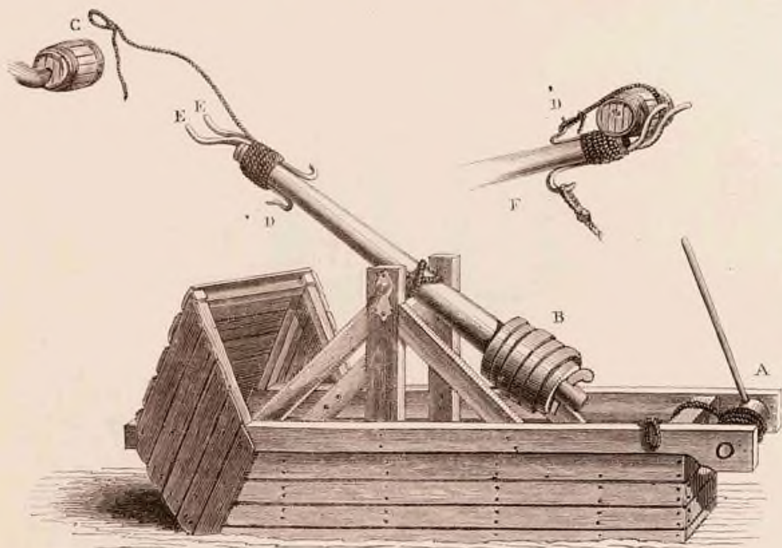
Fig. 66. — Bricole. — La force centrifuge, quand le style pivote rapidement sur son axe, fait échapper l'œil C du crochet D; alors le barillet, dirigé par la fourche EE, s'échappe et est projeté au loin. — F, bout du style, lorsqu'il est abaissé par le treuil A et chargé de son baril de feu ou de fer. — B, rondelles de pierre, de fer ou de plomb.
