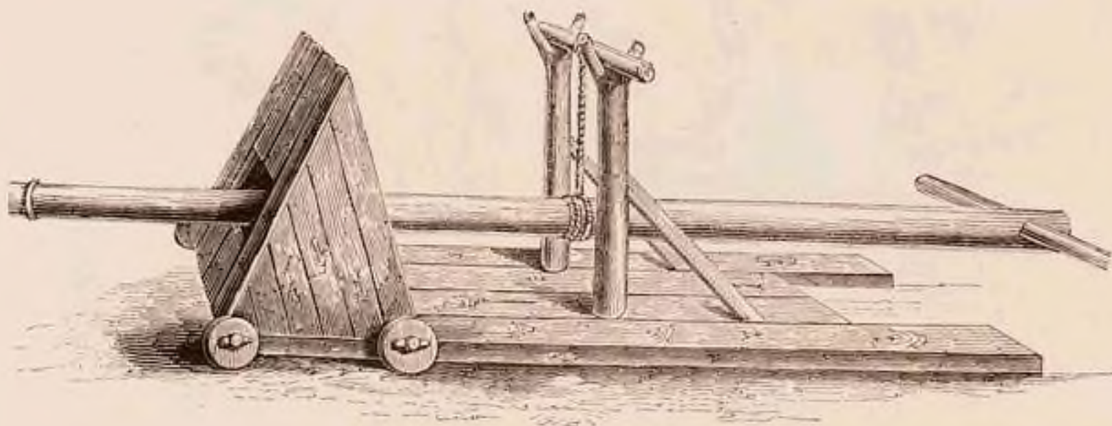
Fig. 65. — Bélier, d'après une miniature du manuscrit 17,339 de la Bibl. nat. de Paris.
